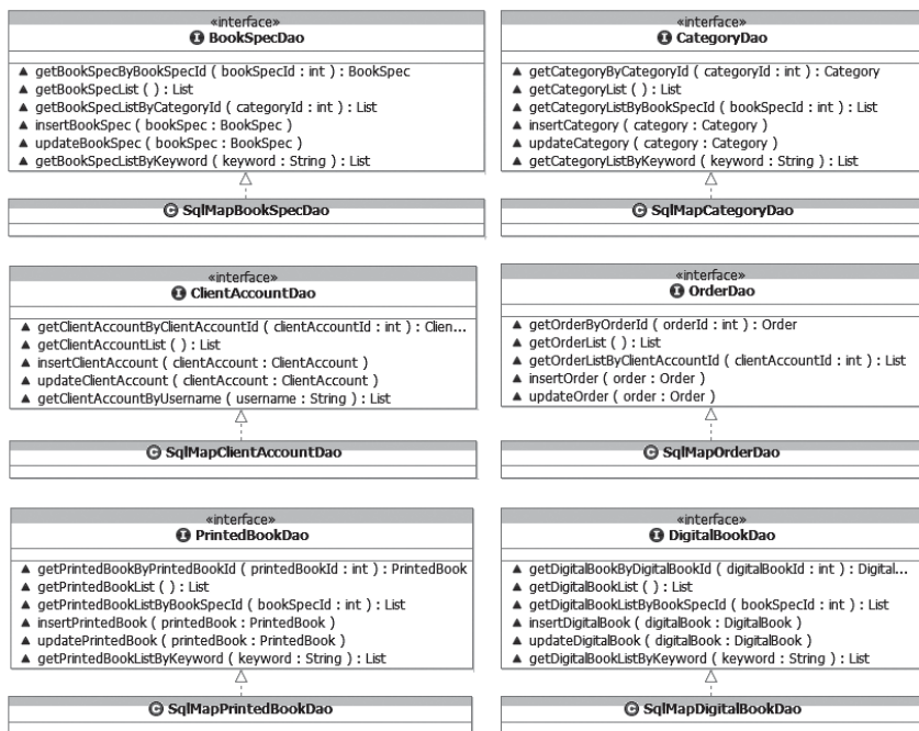
Figura 5-12. PSM Java: puente entre el modelo relacional y el modelo de dominio. Interfaces.
